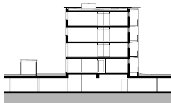
SCHNITT - HAUS E
