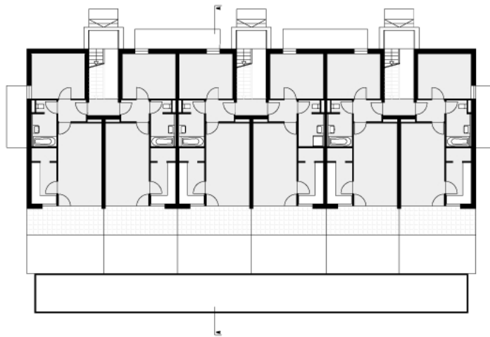
ERDGESCHOSS - HAUS A
