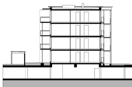
SCHNITT - HAUS C
