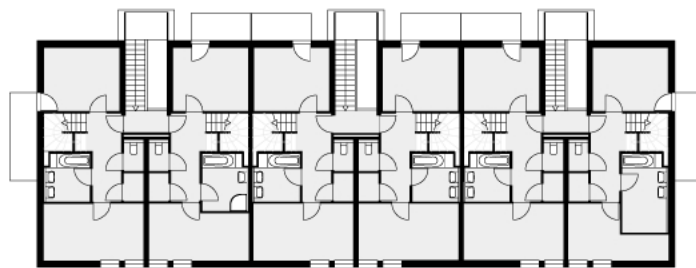
1. OBERGESCHOSS - HAUS A
