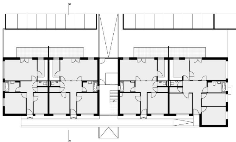
ERDGESCHOSS - HAUS C
